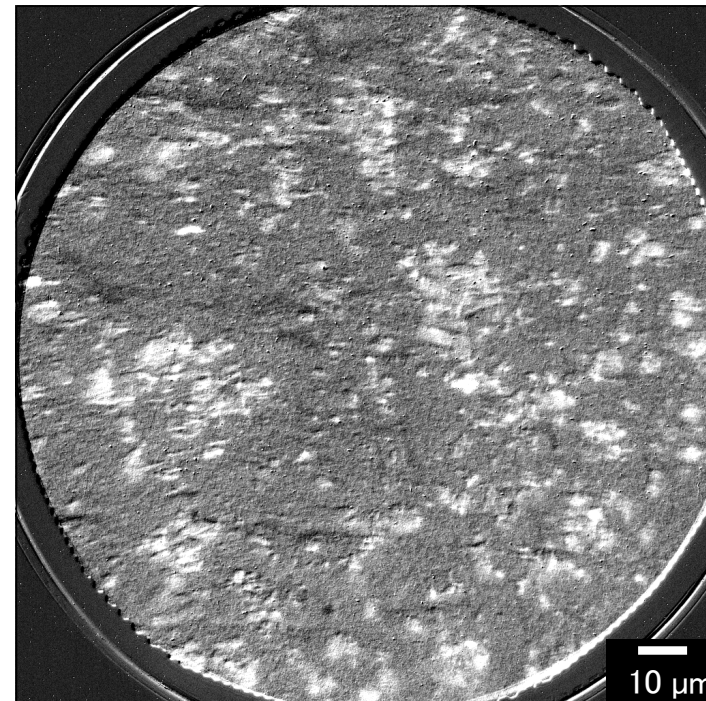
液体リチウムイオン電池用電極表面のLiの分布像
